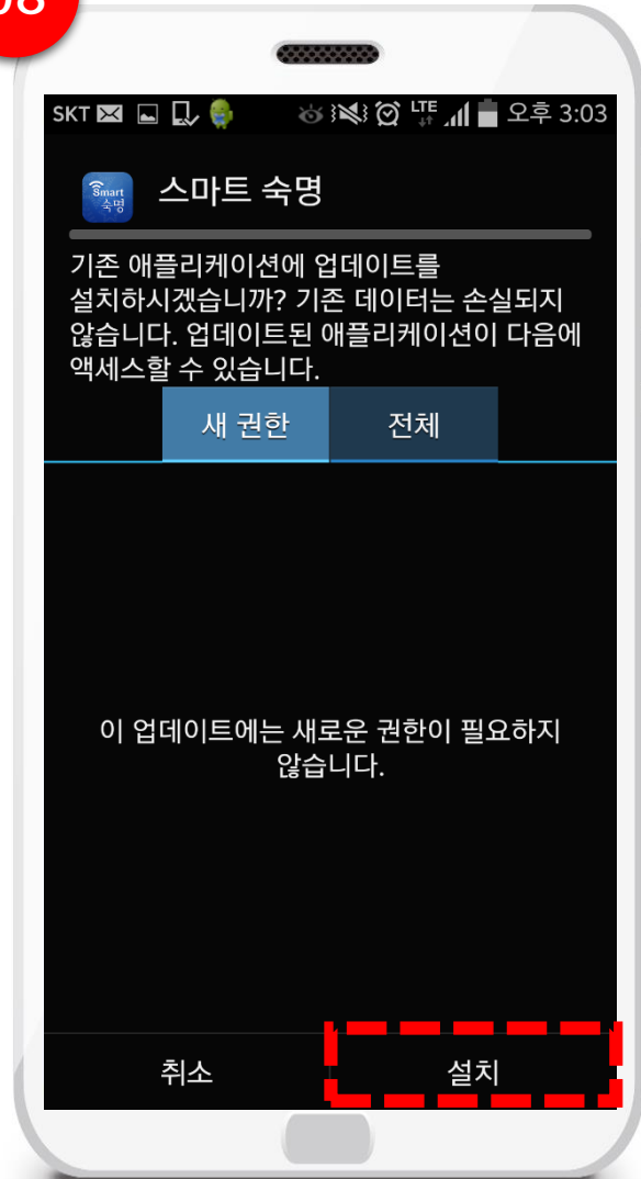
[권한설정]에서 [설치]탭!
