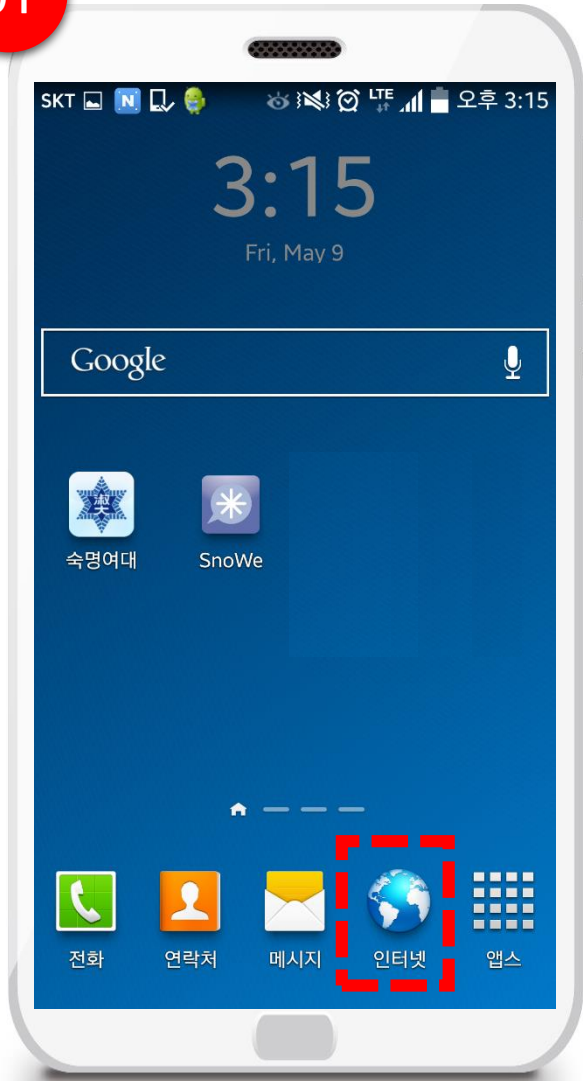
인터넷 실행
