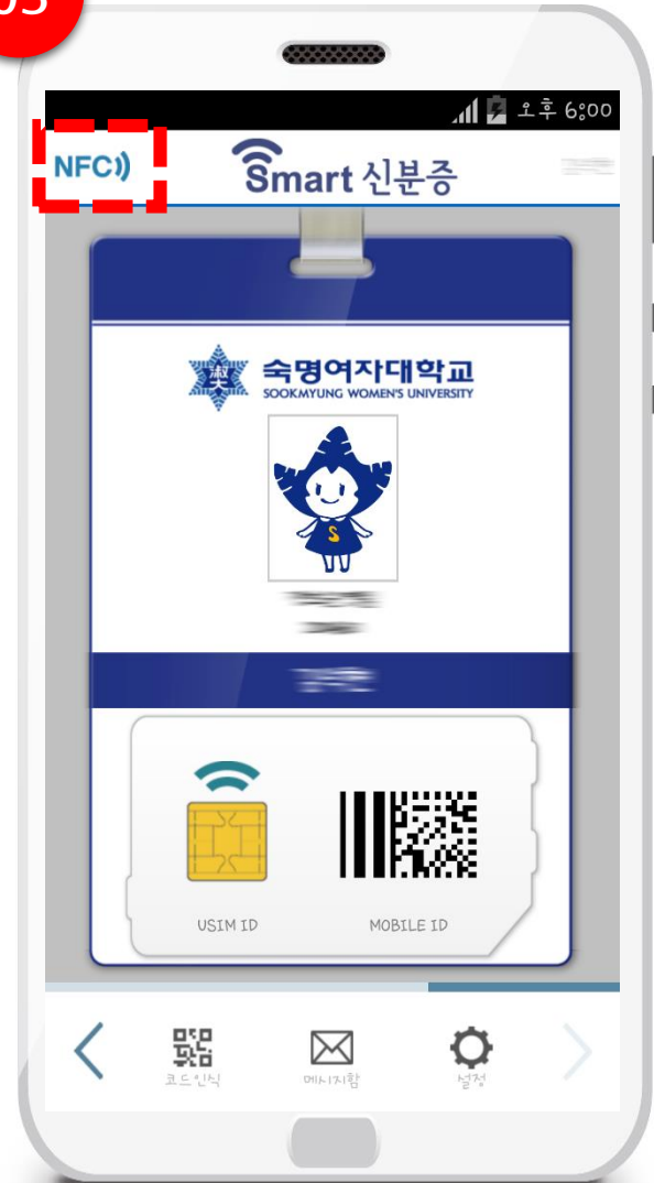
활성화 확인
